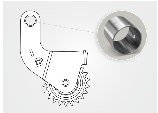
Asiento en tensor de cadena con casquillo de cojinete PERMAGLIDE® P200/P201
