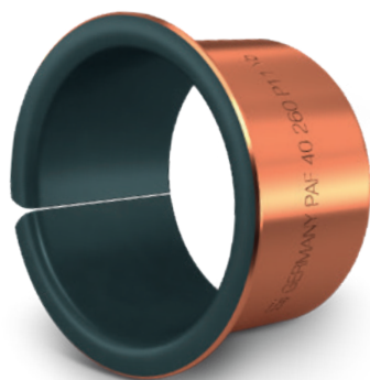
Casquillos con collarín PERMAGLIDE® del tipo de construcción PAF... P11
