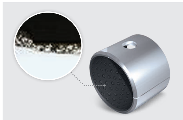
Fig. 22: Cojinetes P20 con bolsas de lubricante y agujero de engrase
