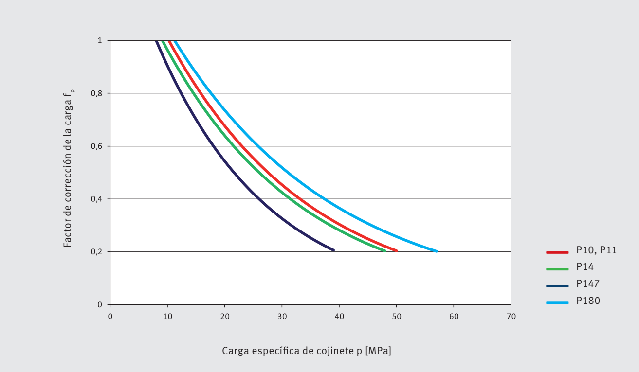
Fig. 25: Factor de corrección de la carga f_p
