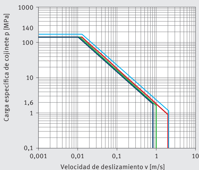
Fig. 10: Valor pv [MPa · m/s], curva límite (valores válidos a temperatura ambiente)
