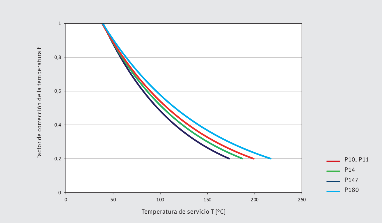
Fig. 26: Factor de corrección de la temperatura f_T
