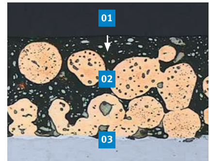
Fig. 2: Sistema de capas P1 01 Lubricante sólido 02 Capa de deslizamiento de bronce 03 Dorso del cojinete
