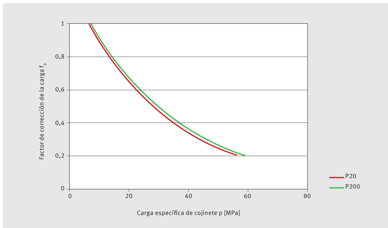
Fig. 29: Factor de corrección de la carga f_p
