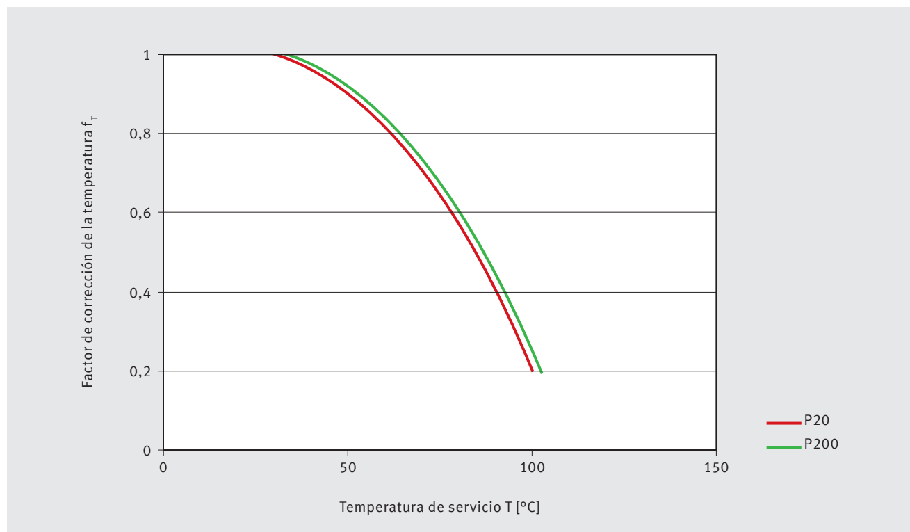
Fig. 30: Factor de corrección de la temperatura f_T
