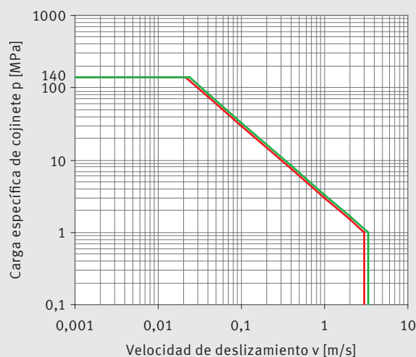
Fig. 14: Valores pv, curvas límite P20, P200 engrasadas a 20 °C
