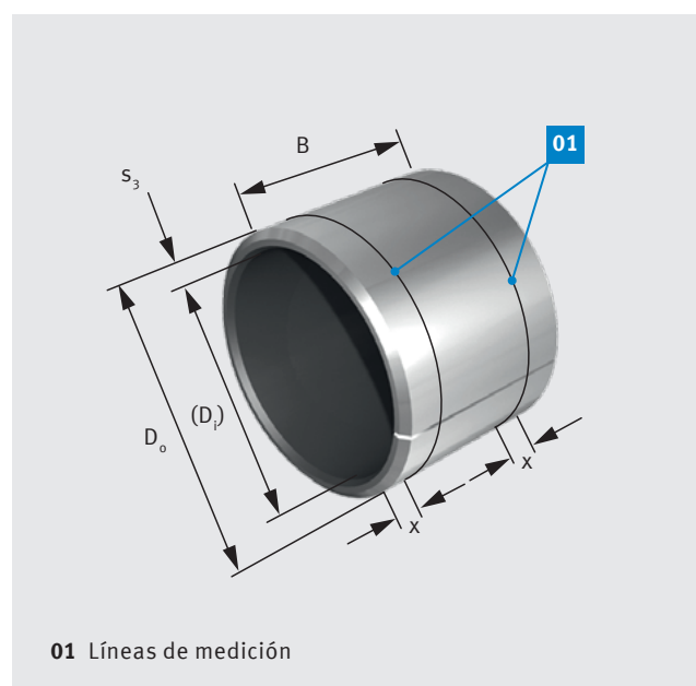
Fig. 66: Líneas de medición para la comprobación del espesor de la pared (ejemplo)
