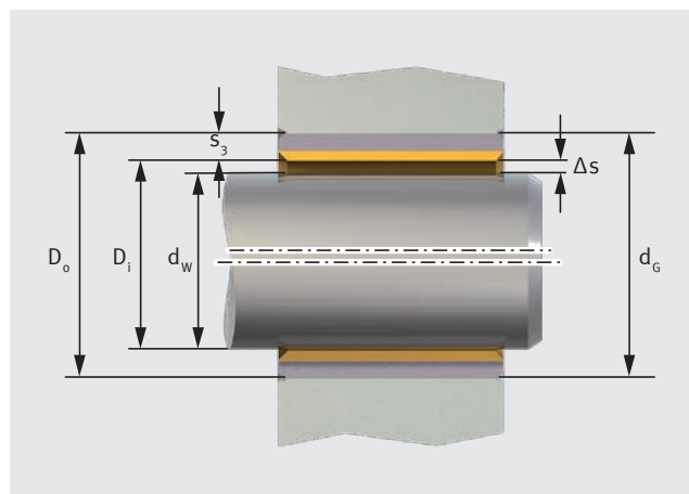
Fig. 50: Holgura teórica del cojinete \Delta s
