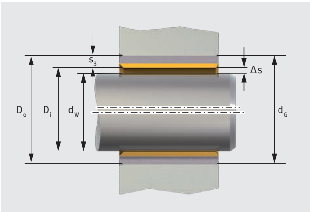
Fig. 48: Holgura teórica del cojinete Δs
