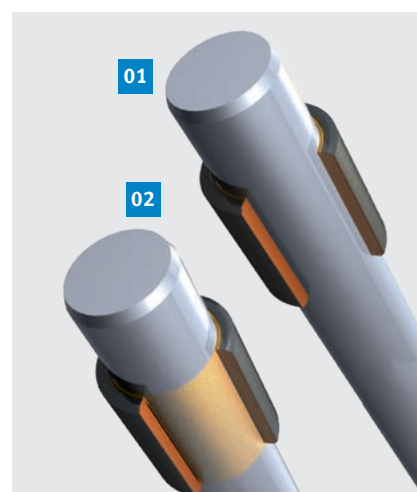
Fig. 6: Transferencia de material
