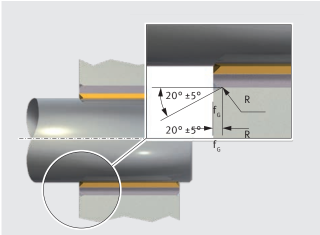
Fig. 40: Bisel en la carcasa para camisa PAP
