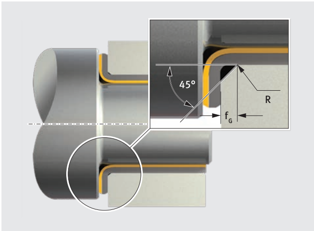
Fig. 41: Bisel en la carcasa para camisa PAF
