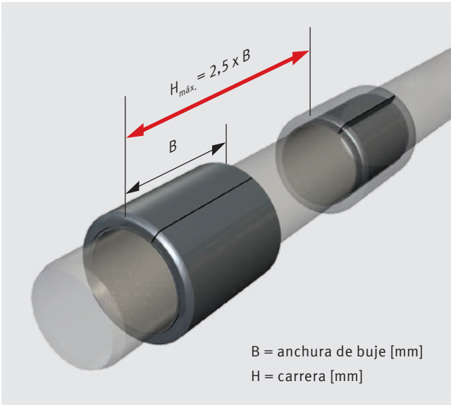
Fig. 34: Movimiento lineal, carrera H_{máx.}
