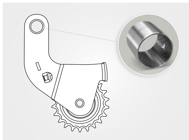
Supporto del tendicatena con boccola a strisciamento PERMAGLIDE® P200/P201
