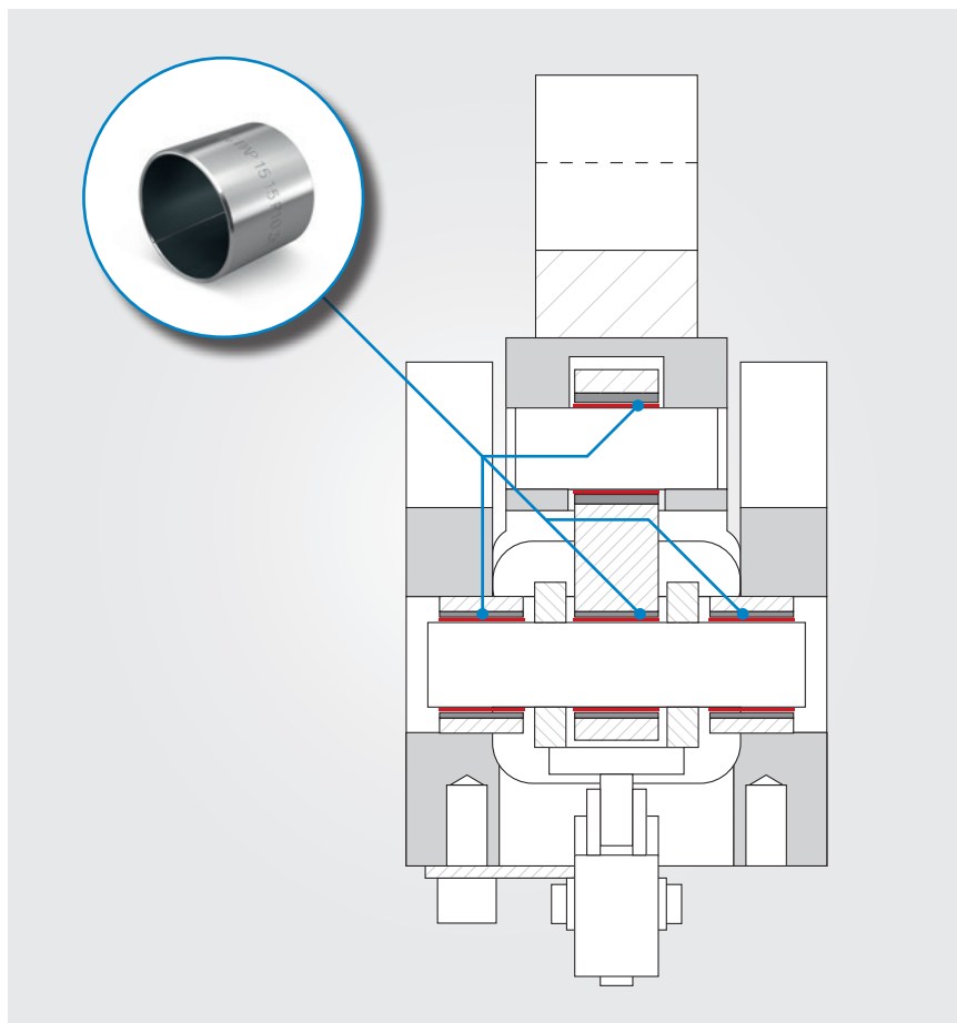
Cuscinetti del perno di articolazione negli attrezzi di fissaggio con leva articolata con boccole a strisciamento PERMAGLIDE® della forma costruttiva PAS ... P10
