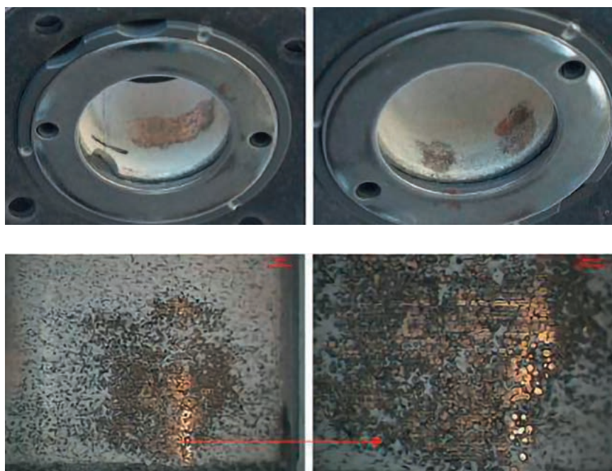
Rys. 39: Znaczne lokalne uszkodzenie spowodowane przez błędy montażu
