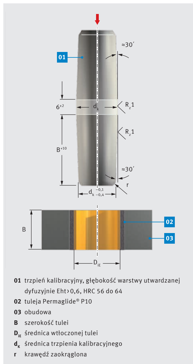
Rys. 55: Kalibracja
