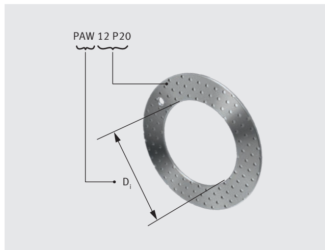
Rys. 64: Przykład zamówienia, podkładka oporowa P20
