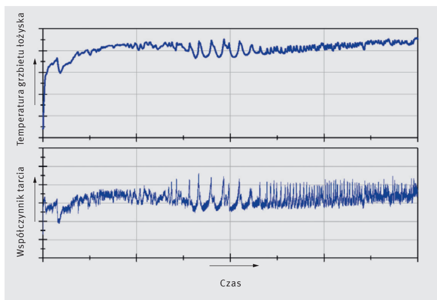
Rys. 7: Wahania współczynnika tarcia i temperatury
