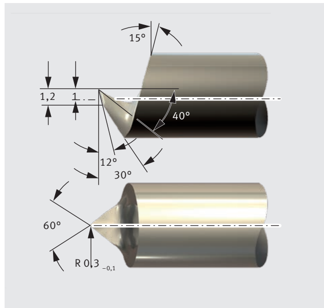
Rys. 67: Narzędzie skrawające do łożysk z materiałów Permaglide® P22 i P202
