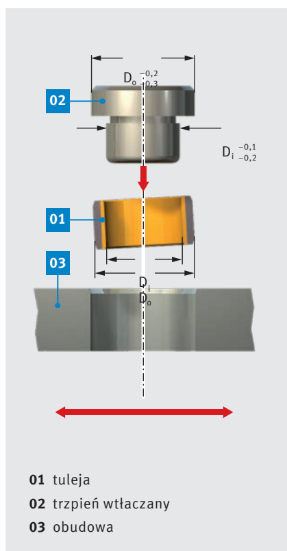
Rys. 51: Wtłaczanie z użyciem ruchomej obudowy
