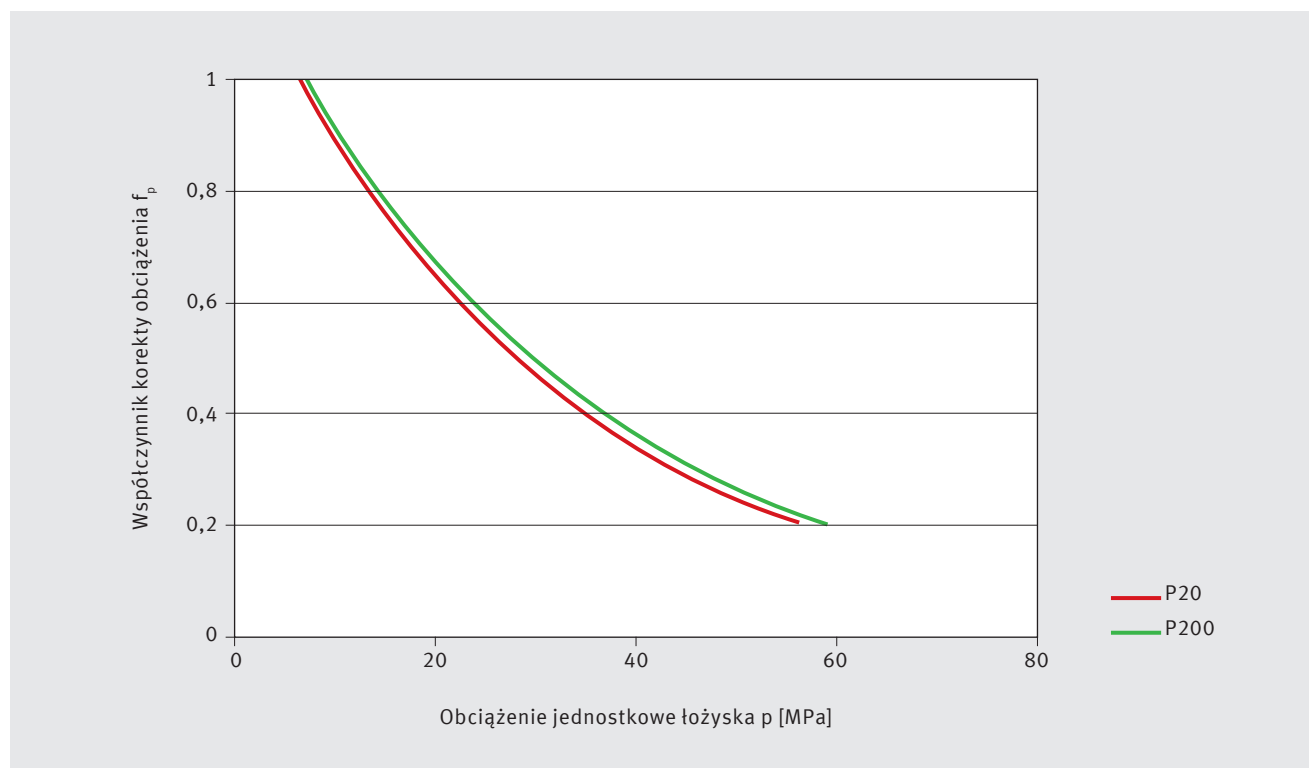
Rys. 29: Współczynnik korekty obciążenia f_p
