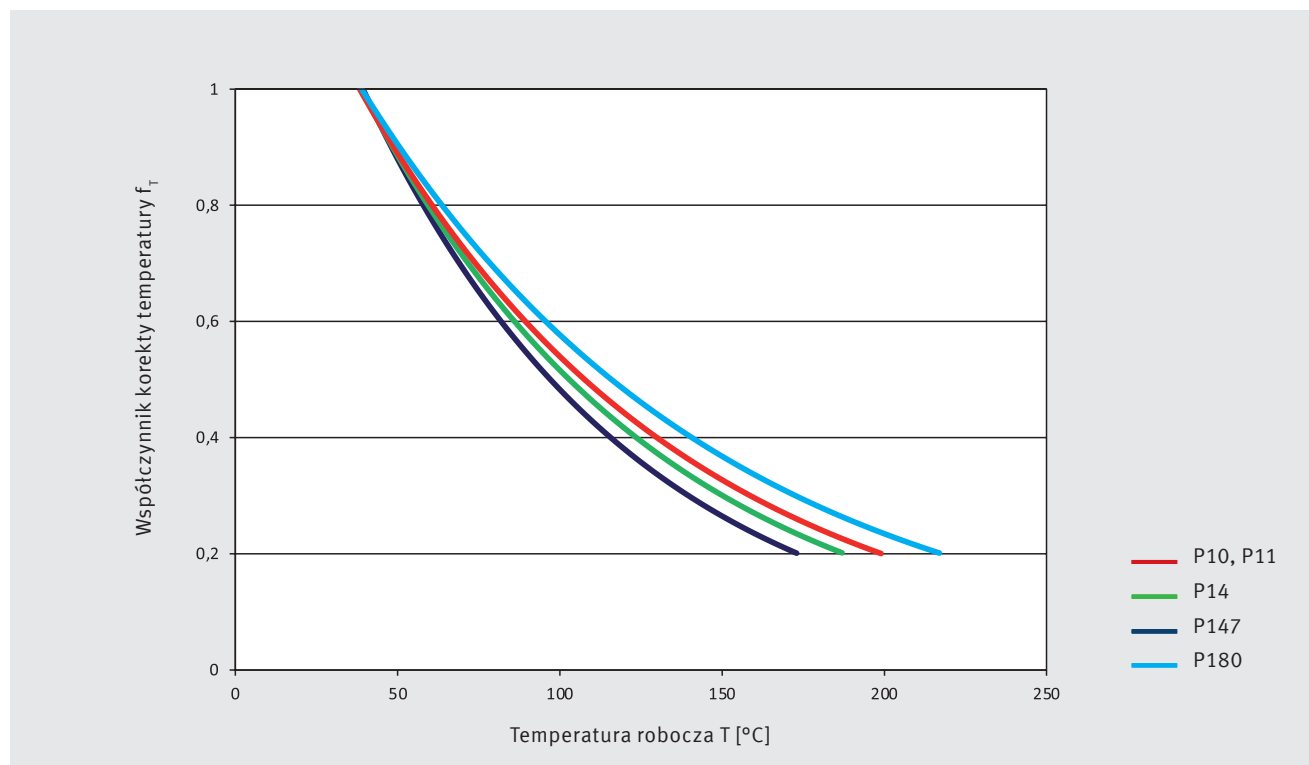
Rys. 26: Współczynnik korekty temperatury f_T
