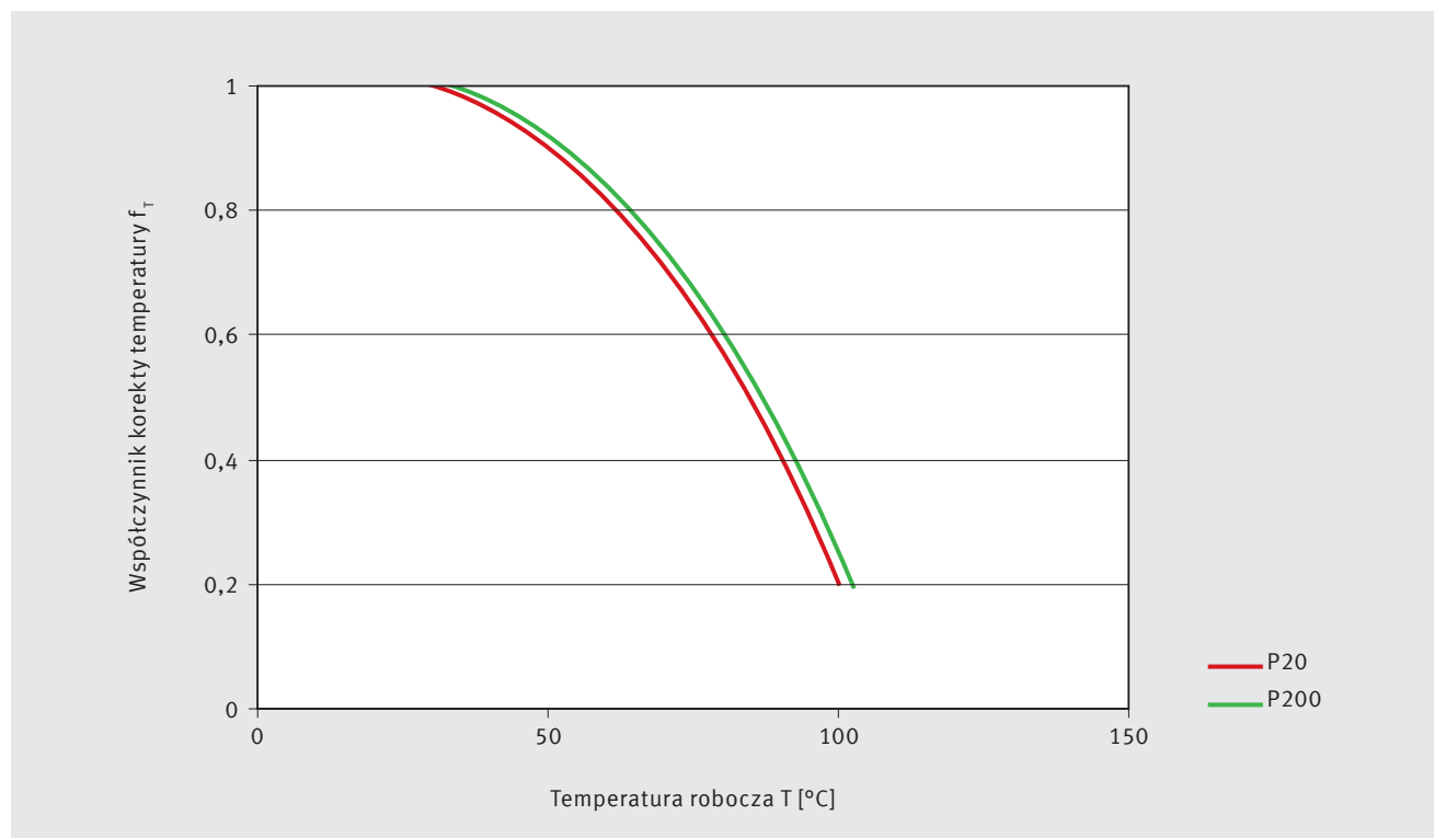
Rys. 30: Współczynnik korekty temperatury f_T
