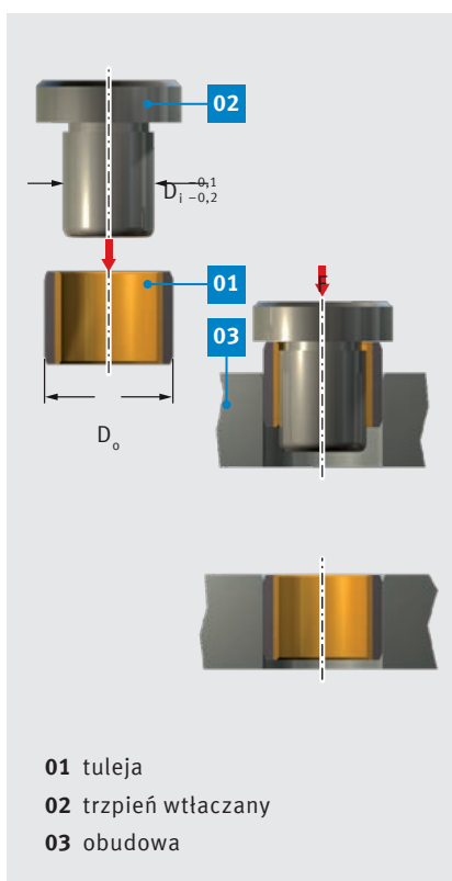
Rys. 52: Wtłaczanie styczne z powierzchnią D_0 \leq 55 mm
