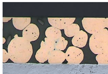
Rys. 8: Właściwości powierzchni ślizgowej w okresie eksploatacji
