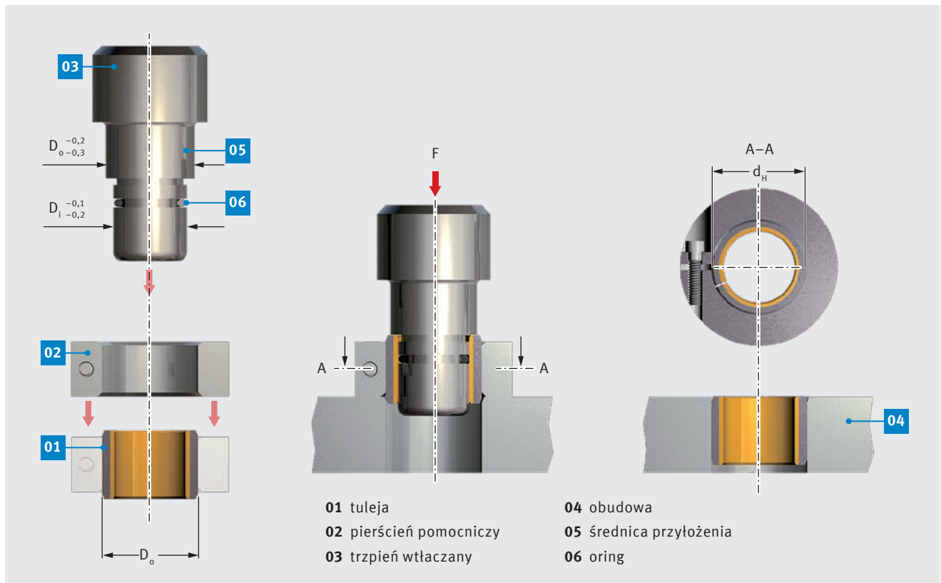
Rys. 54: Wślaczanie tulei, D_o \geq 55 mm, przy użyciu pierścienia montażowego
