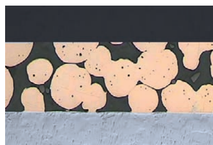
Rys. 9: Właściwości powierzchni ślizgowej na końcu okresu eksploatacji
