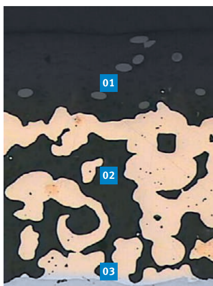
Rys. 12: System warstw P2
