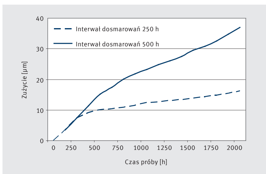
Rys. 13: Charakterystyka zużycia łożysk ślizgowych P2 (schemat)
