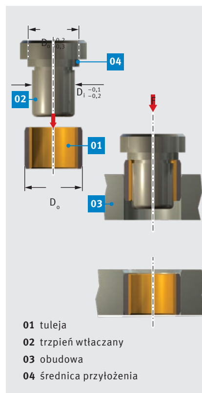
Rys. 53: Wtłaczanie obniżone D_0 \leq 55 mm
