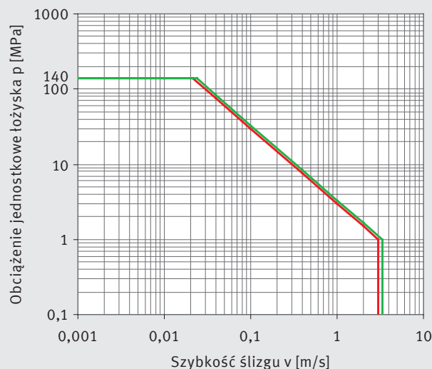
Rys. 14: Wartości p_v , wykresy graniczne P20, P200, smarowanie smarem przy temperaturze 20 °C
