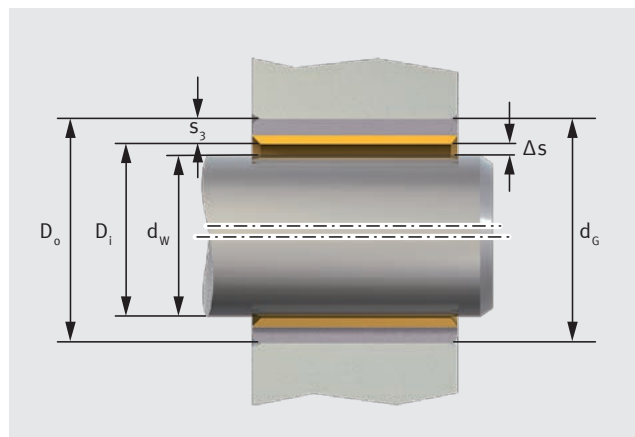
Rys. 48: Teoretyczny luz łożyskowy \Delta s
