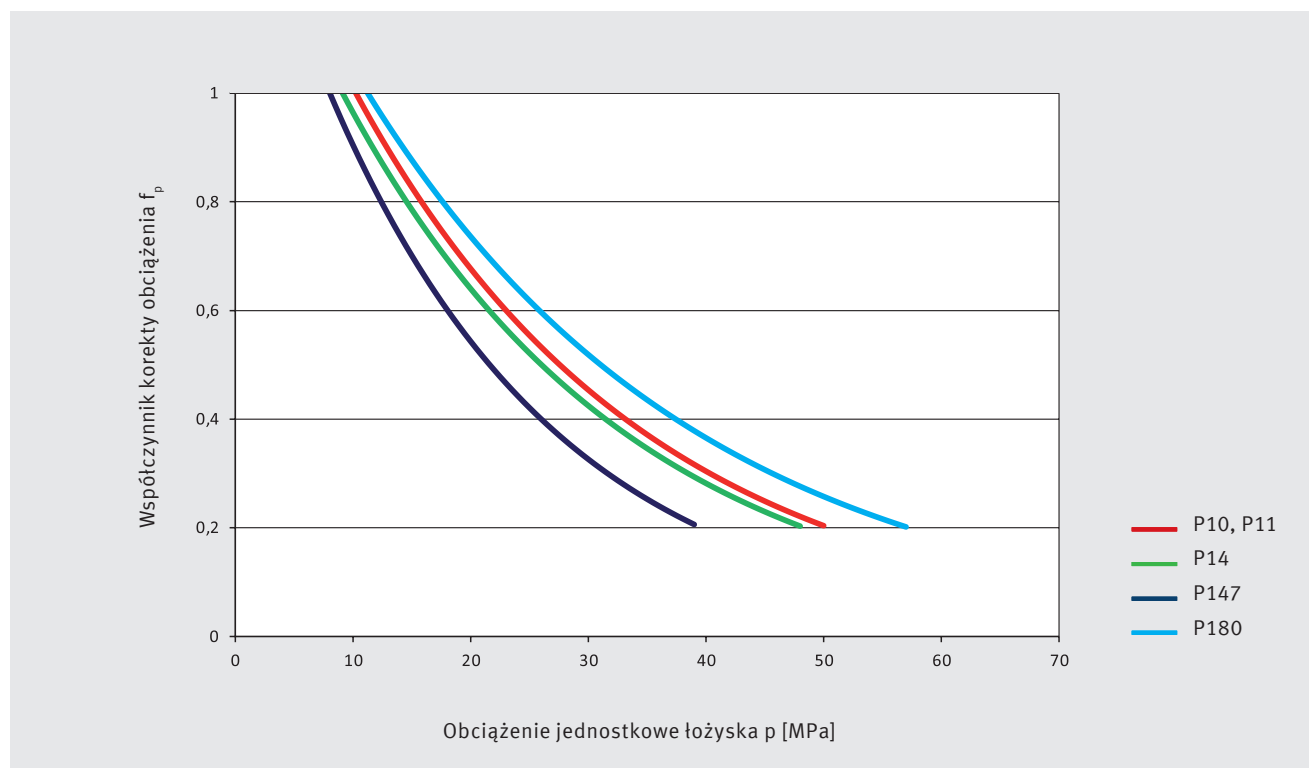
Rys. 25: Współczynnik korekty obciążenia f_p
