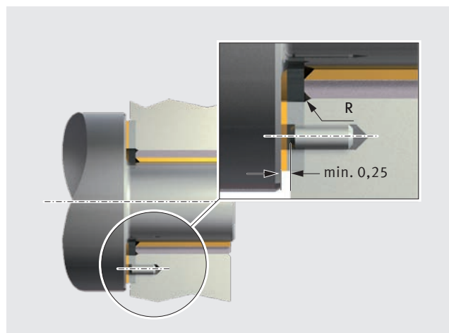
Rys. 42: Mocowanie podkładki oporowej PAW w wyfrezowaniu obudowy
